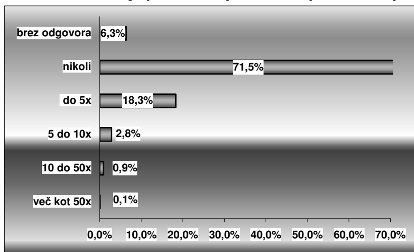
Graf 3.6.2.3: Metanje predmetov (frekvenčna porazdelitev)
